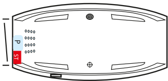
LOTUS 1900 – Gesamthöhe 59-62 cm
