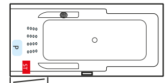
CAMA 1900 rechts – Gesamthöhe 58-61 cm
