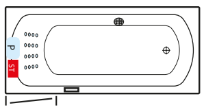
OBJEKT 1800 – Gesamthöhe 57-60 cm
