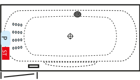
BOA 1800 – Gesamthöhe 59-62 cm
