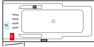
CAMA 2000 rechts – Gesamthöhe 58-61 cm
